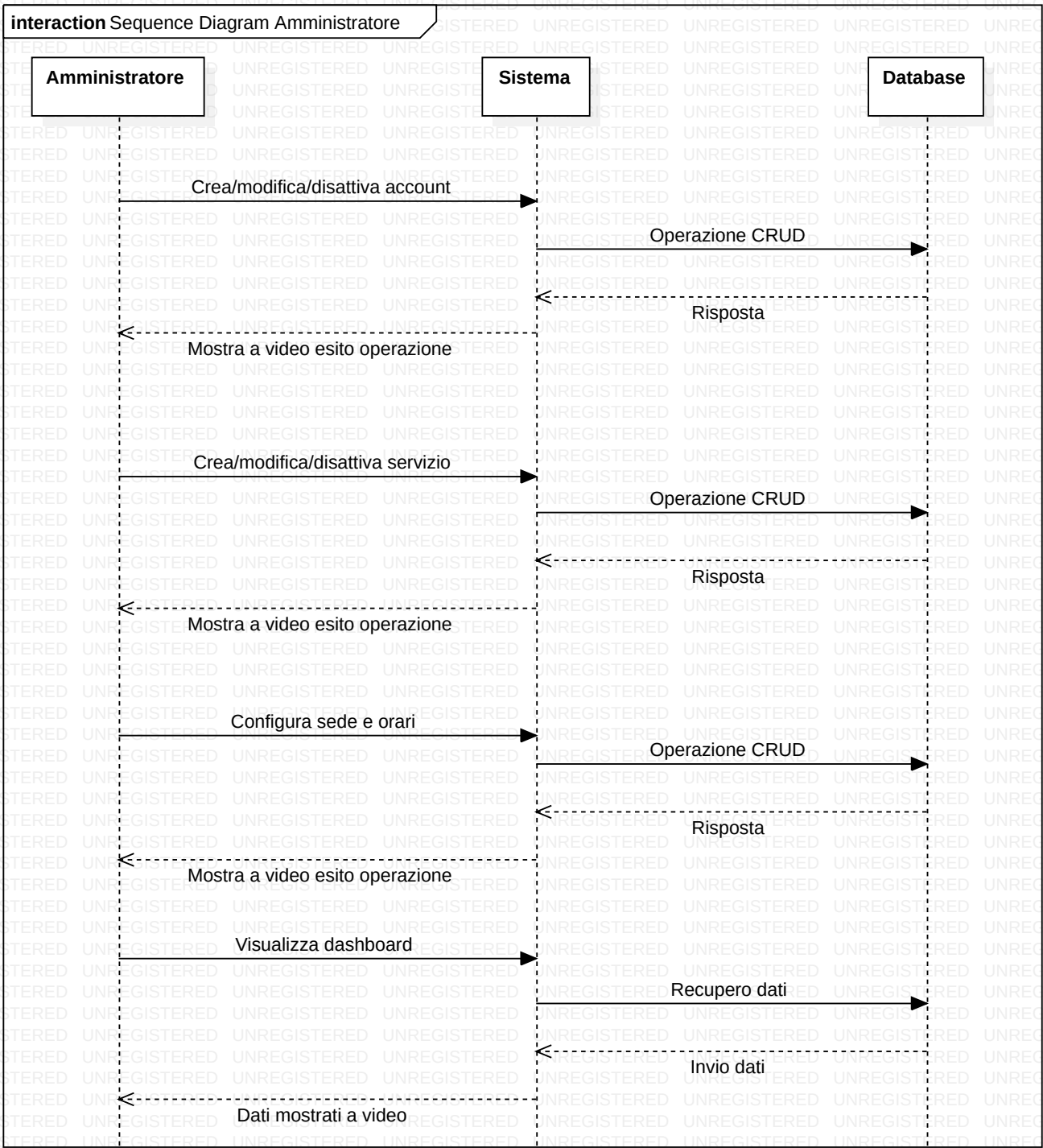
Diagramma a Sequenza Diagram Amministratore
